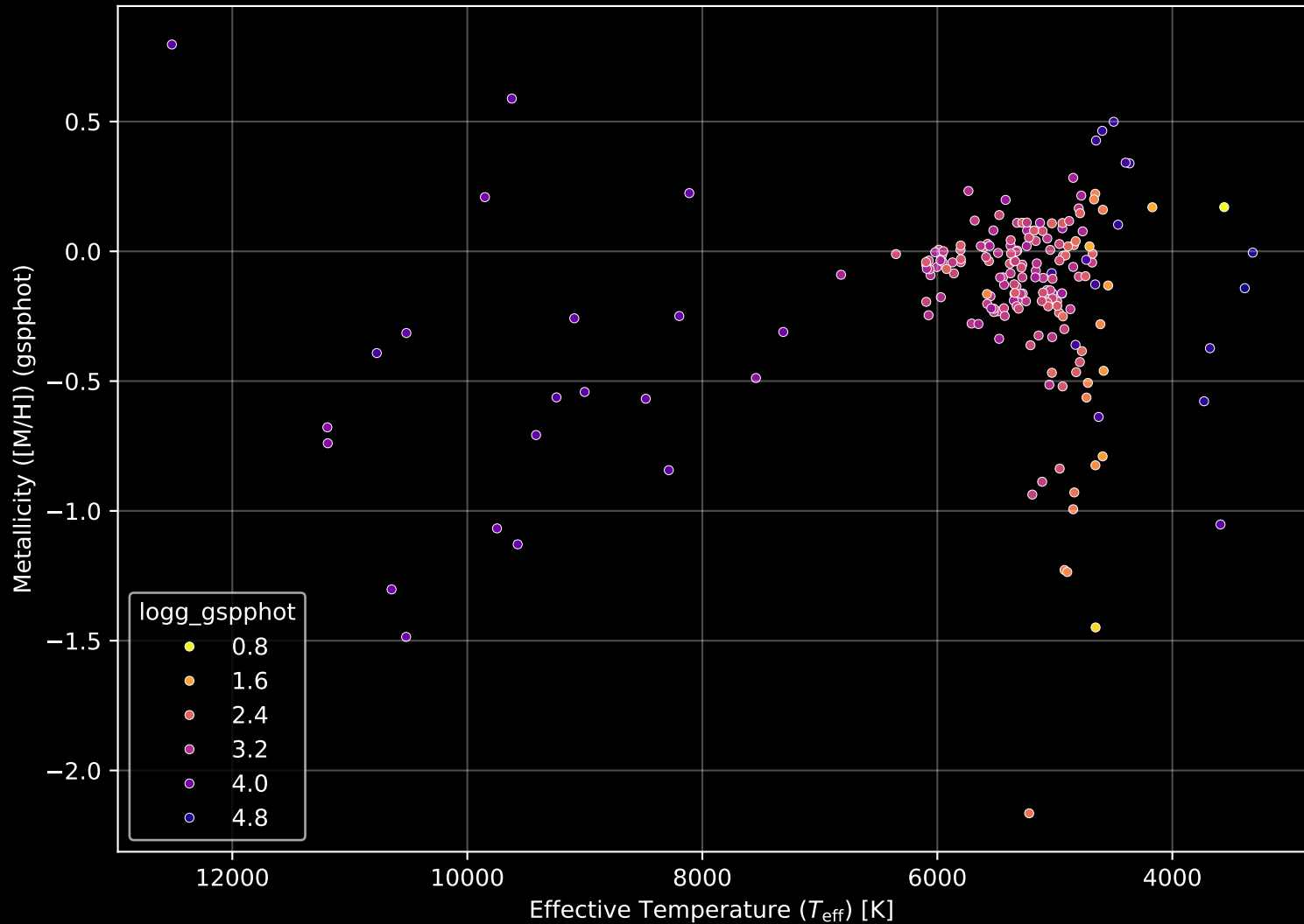
APOGEE DR17 Field: [158+04] Stellar Population Parameters (n= 200)
